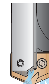
Hűtőcsatorna-rendszer 4 kilépési furattal
