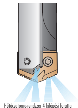
Hűtőcsatorna-rendszer 4 kilépési furattal
