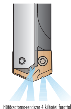
Hűtőcsatorna-rendszer 4 kilépési furattal
