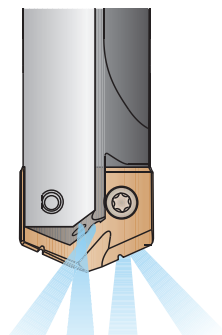
Hűtőcsatorna-rendszer 4 kilépési furattal
