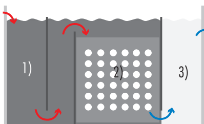
Idegen olajok kivezetése szinteltoltó tartályba (túlfolyás elleni védelem)
