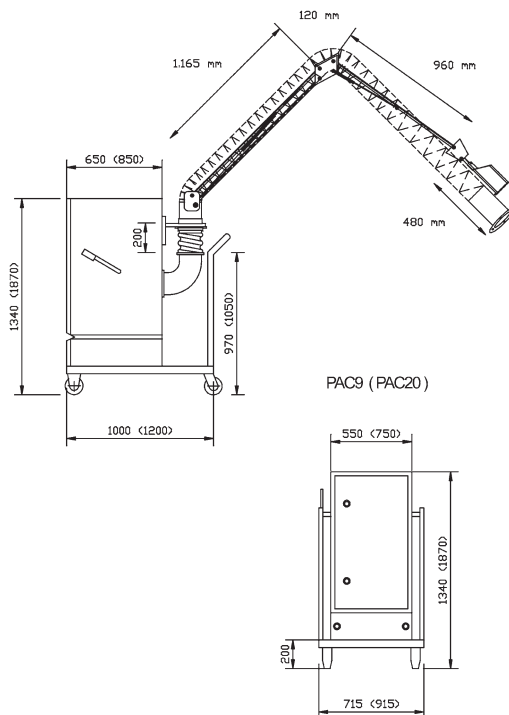
Az ábra a SARA-PAC 20-at mutatja porgyűjtő váddal és utánszűrővel
