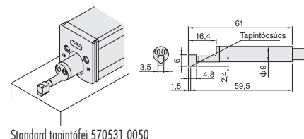
Standard tapintófej 570531 0050
