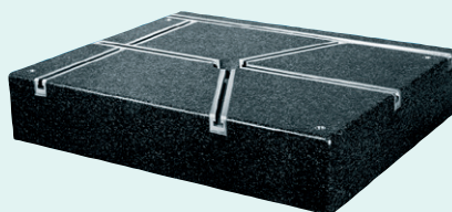
Keménycőzet lemez 5 T-horonsínnel (különleges kivitel)
