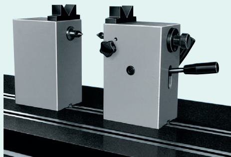
Szegnyeregpár lemezen T-horonsínekkel
