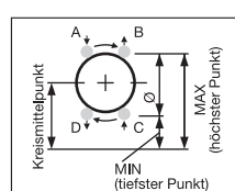
Kör, furat és tengely mérése
