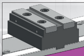
Lépcsős közbenső befogó (2+3) cserélhető befogó betéttel
