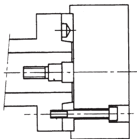
közvetlen tokmányfelfogatás
