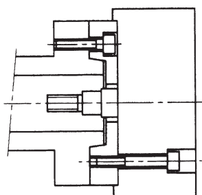
közvetett tokmányfelfogatás
